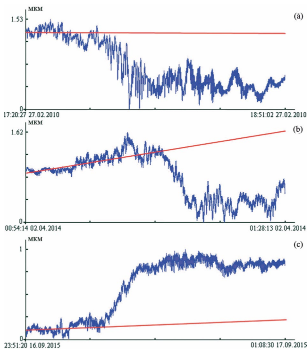
Рис. 4. Фрагменты записей 52,5-метрового лазерного деформографа: а – февраль 2010 г., б – апрель 2014 г., с – сентябрь 2015 г.
